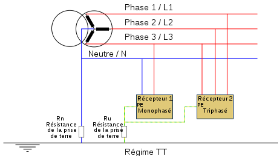
Exemple d'un schéma de liaison à la terre TT
